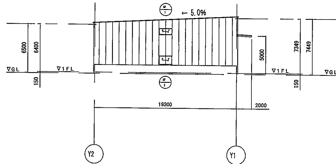
X1通り立面図
