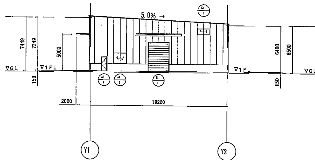
X6通り立面図
