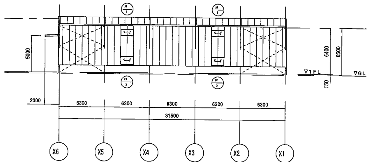
Y2通り立面図
